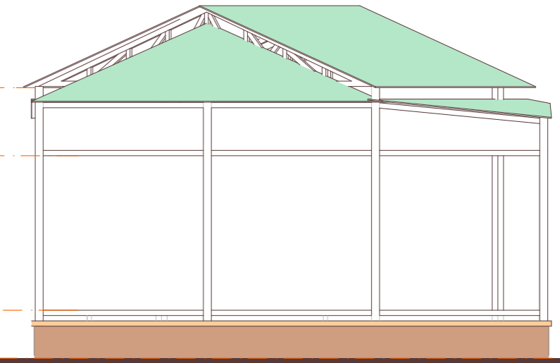
Вид 2-2 М 1;100
